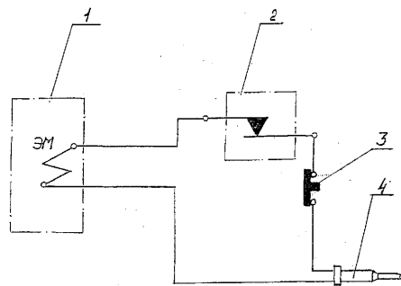
1 - блок автоматики; 2 - датчик тяги; 3 - кнопка аварийная; 4 - термopapa.
